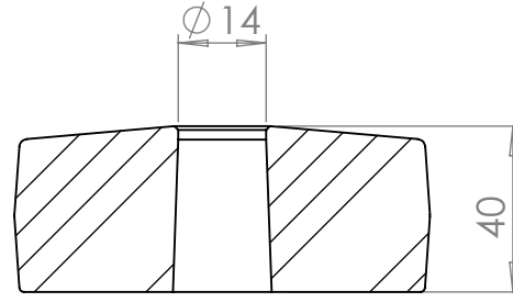
KESİT D-D
