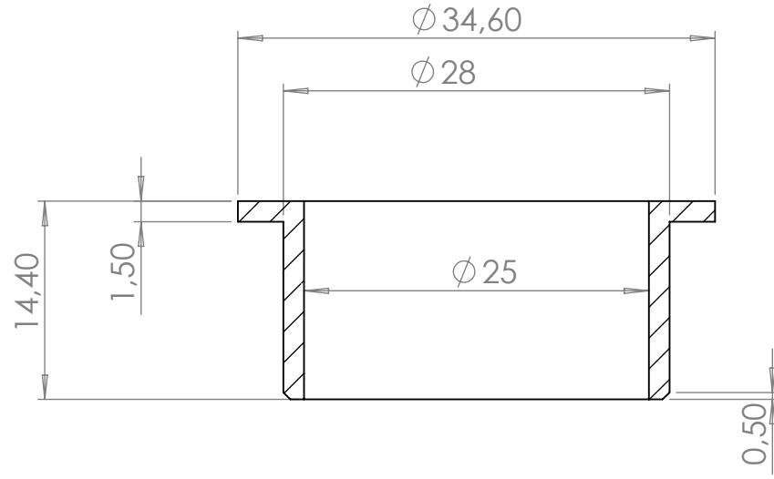
KESİT A-A
